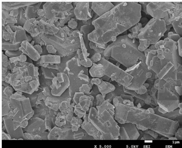
ZSM-5 SEM
